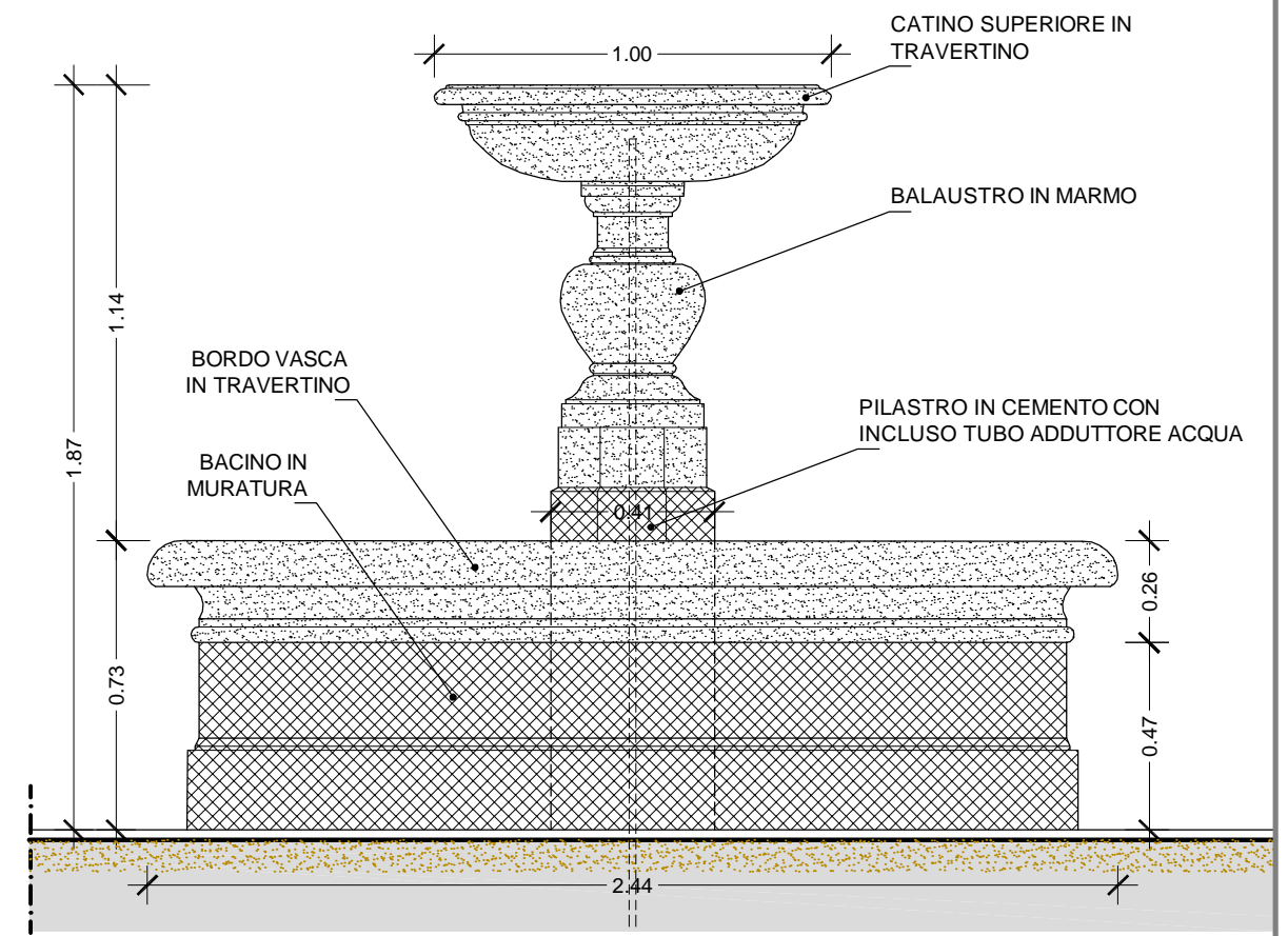
PROSPETTO
